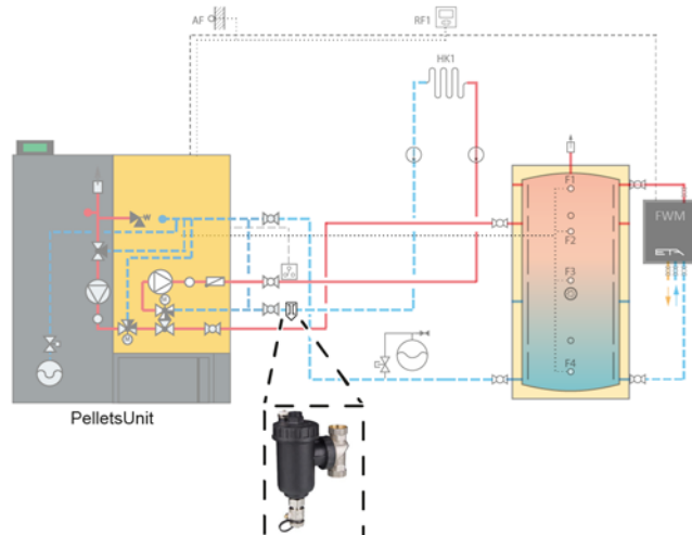
Fig. 7-7: Position d'installation pour chaudières avec circuit de chauffage intégré
