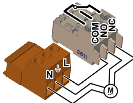
Fig. 11-7: Fonction spéciale - Vanne de commutation avec commande à 3 points
