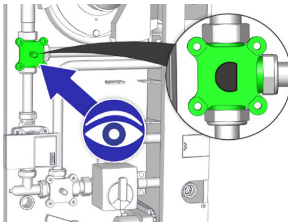
Fig. 10-14: Mélangeur de départ
