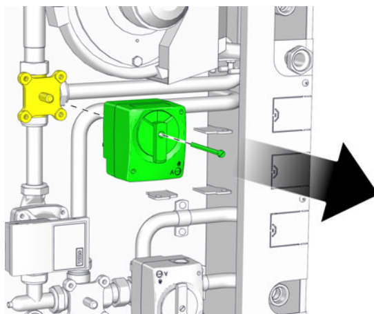
Fig. 10-13: Servomoteur au niveau du mélangeur de départ
