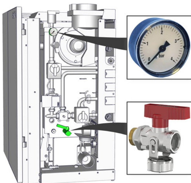
Fig. 10-23: Manomètre, robinet de remplissage et de purge
