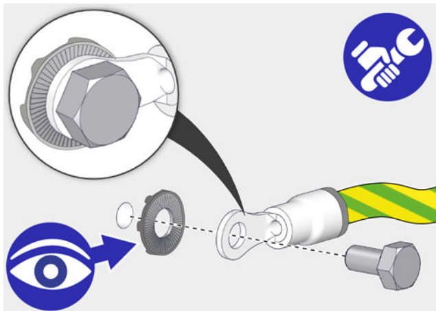
Fig. 11-1: Rondelle de contact
