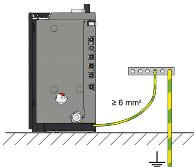
Fig. 10-22: Raccorder la liaison équipotentielle
