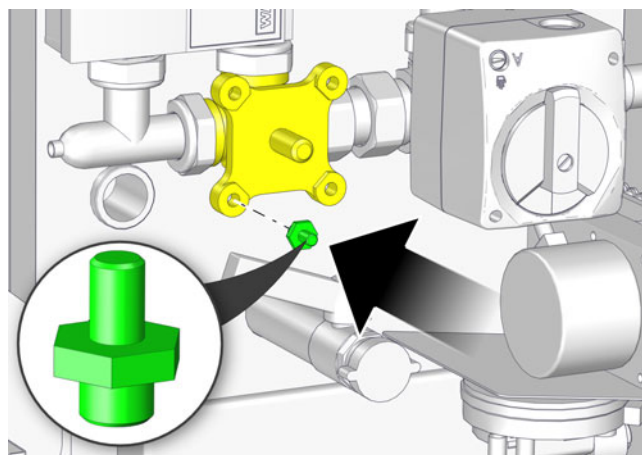
Fig. 10-16: Dispositif de fixation
