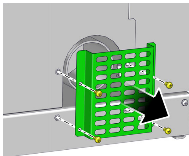
Fig. 10-3: Grille de protection
