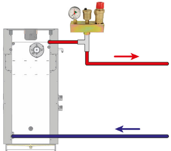
Fig. 7-8: Position correcte de la purge d'air
