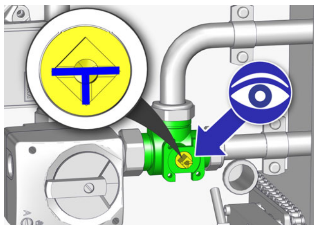
Fig. 10-21: position correcte de la vanne de commutation
