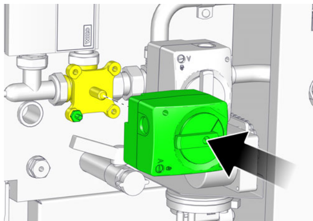
Fig. 10-18: Servomoteur sur la vanne de retour
