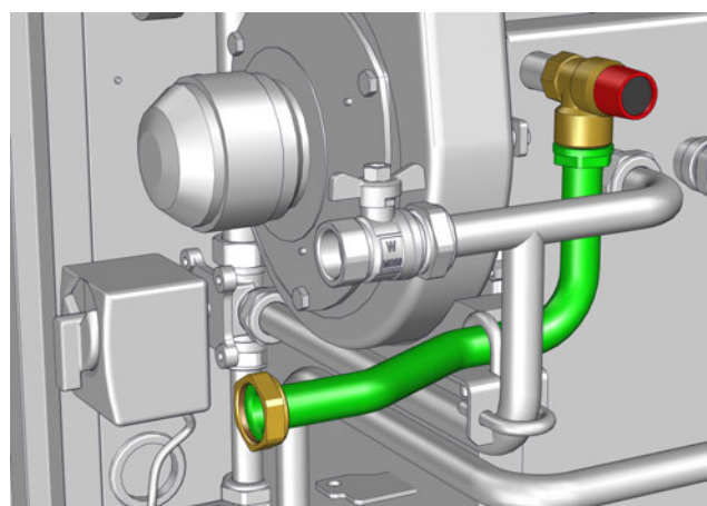
Fig. 10-10: Soupape de sécurité de la chaudière
