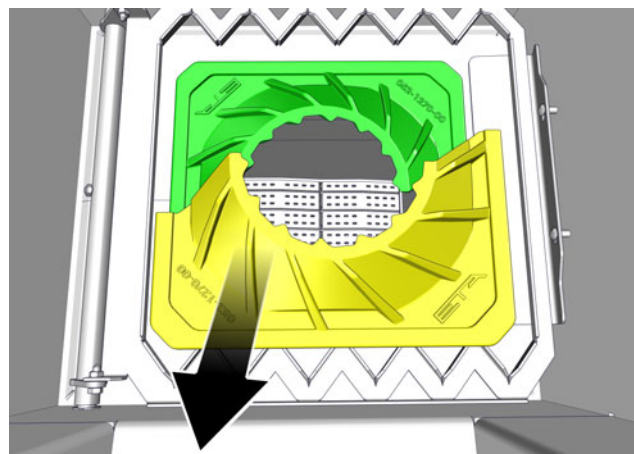
Fig. 6-6: Dépose du couvercle du foyer
