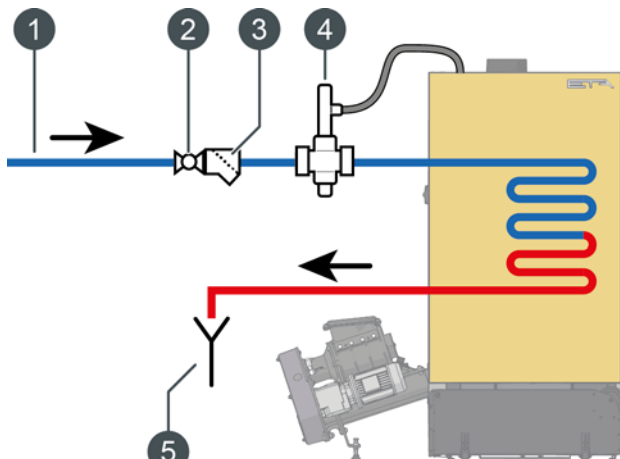
Fig. 3-3: Soupape thermique de sécurité
