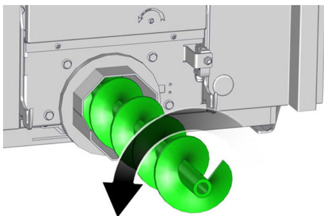
Fig. 6-4: Démontage de la vis d'évacuation des cendres
