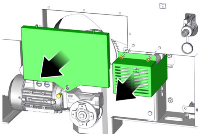
Fig. 6-21: Couvercles
