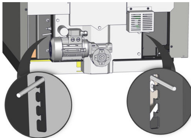
Fig. 2-6: Levier
