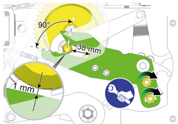
Fig. 6-17: Extraction à droite
