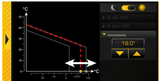
Fig. 5-103: Limite de chauffe pour le mode chauffage
