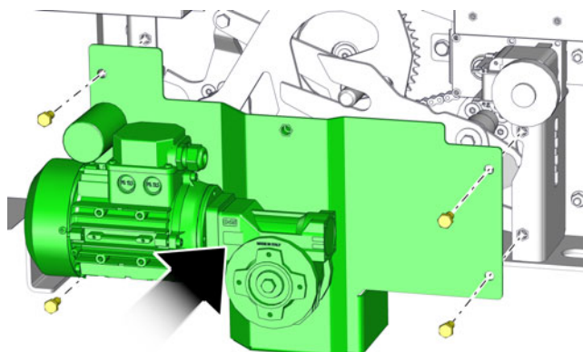
Fig. 6-19: Moteur
