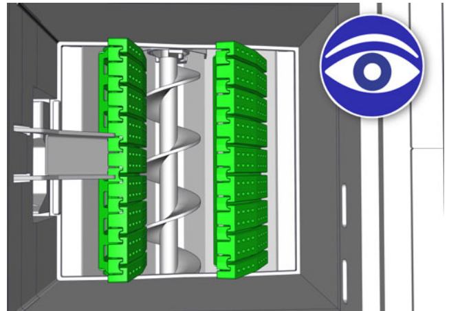
Fig. 6-9: Grille basculante pivotée
