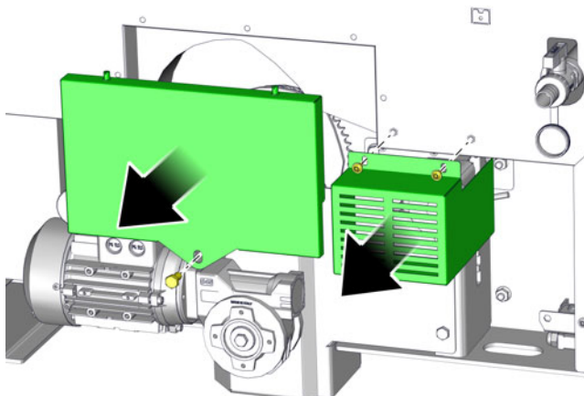
Fig. 6-11: Couvercles
