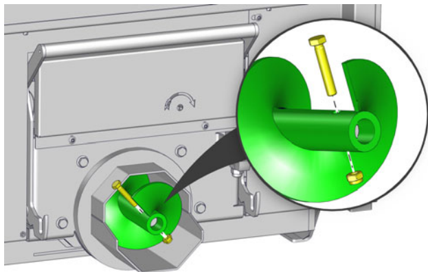
Fig. 6-3: Démontage de la vis
