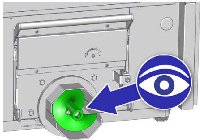
Fig. 6-2: Vis d'évacuation des cendres
