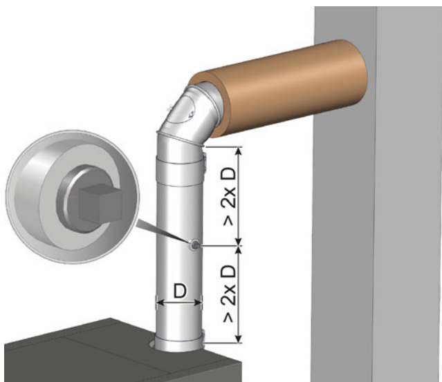
Fig. 8-1: Orifice de mesure
