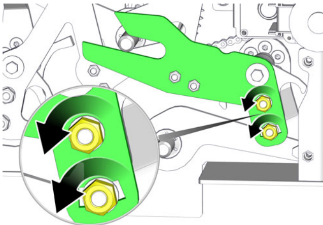
Fig. 6-15: Écrous
