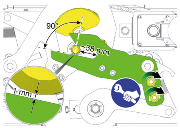
Fig. 6-16: Extraction à gauche
