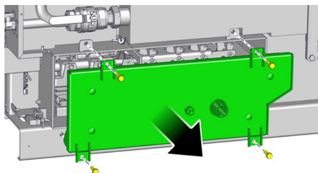
Fig. 6-23: Trappe de visite
