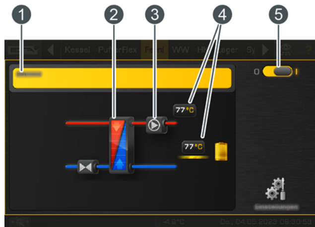
Fig. 5-119: Réseau comme station de transfert
