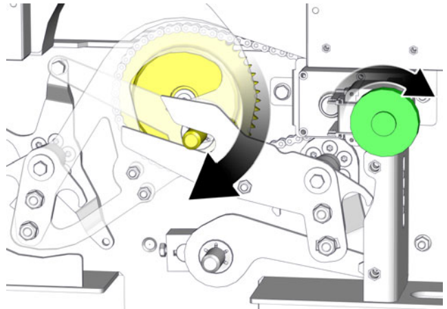
Fig. 6-13: Manivelle
