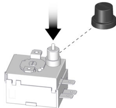
Fig. 3-4: Déverrouiller le contacteur de sécurité thermique
