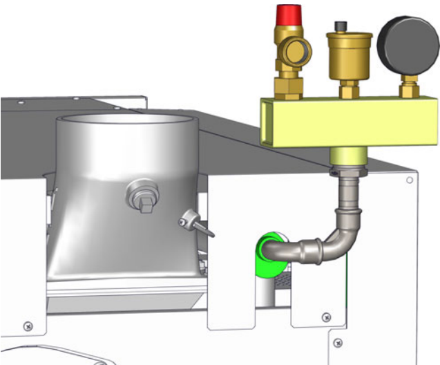
Fig. 3-6: Raccord
