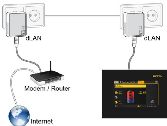
Fig. 5-33: Réseau dLAN
