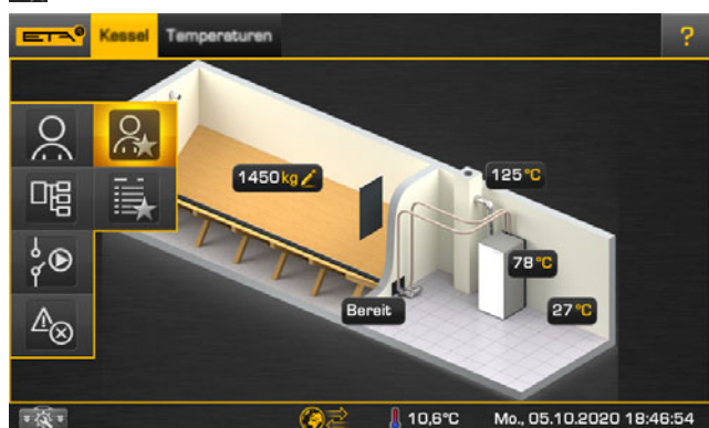
Fig. 5-47: Vue utilisateur
