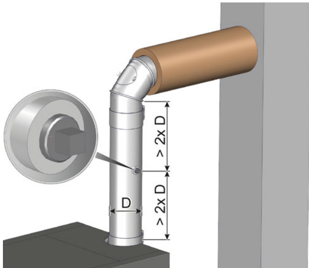
Fig. 6-1: Orifice de mesure
