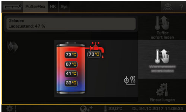
Fig. 5-83: Accumulateur hygiénique
