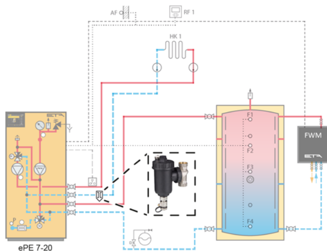
Fig. 8-2: Position d'installation pour chaudières avec circuit de chauffage intégré
