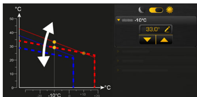
Fig. 5-101: Ajustement de la courbe de chauffage (en cas de températures extérieures inférieures au point de gel)
