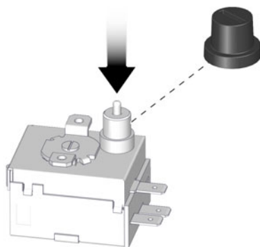
Fig. 3-3: Déverrouiller le contacteur de sécurité thermique
