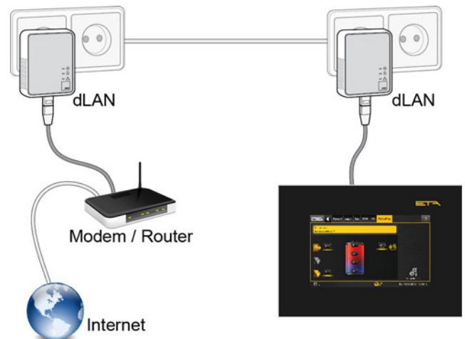
Fig. 5-33: Réseau dLAN
