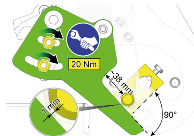
Fig. 8-18: Extraction à gauche
