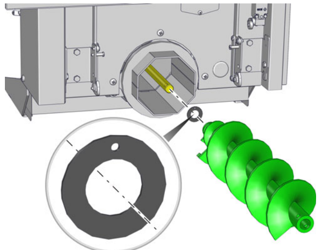
Fig. 8-6: Insertion de la rondelle de glissement
