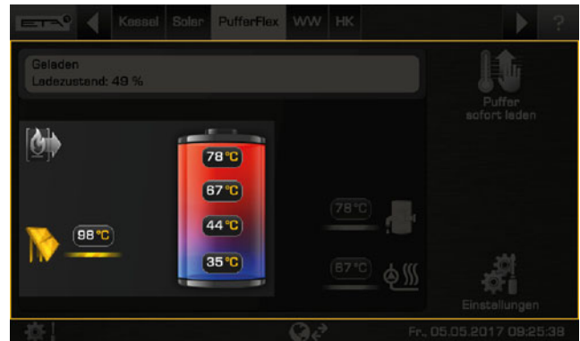
Fig. 6-82: Installation solaire sur le ballon tampon
