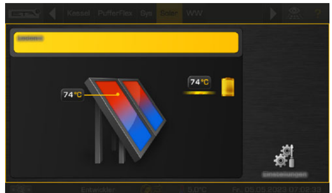
Fig. 6-107: Installation solaire avec commutation entre 2 serpentins dans le ballon tampon
