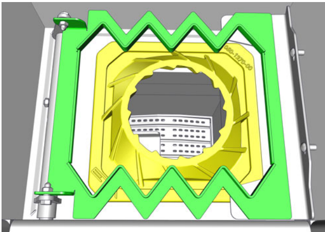
Fig. 8-12: Couvercle du foyer
