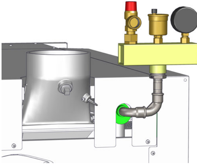
Fig. 3-4: Raccord
