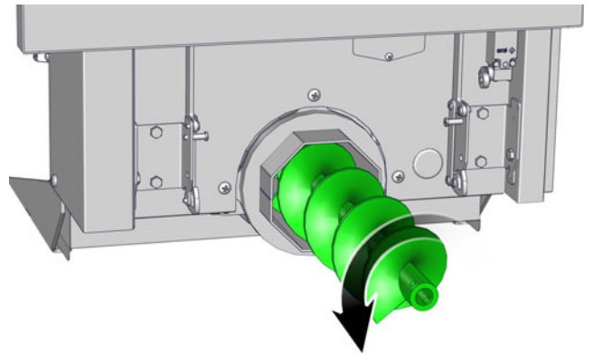
Fig. 8-5: Démontage de la vis d'évacuation des cendres
