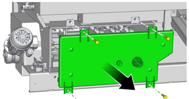
Fig. 8-22: Trappe de visite
