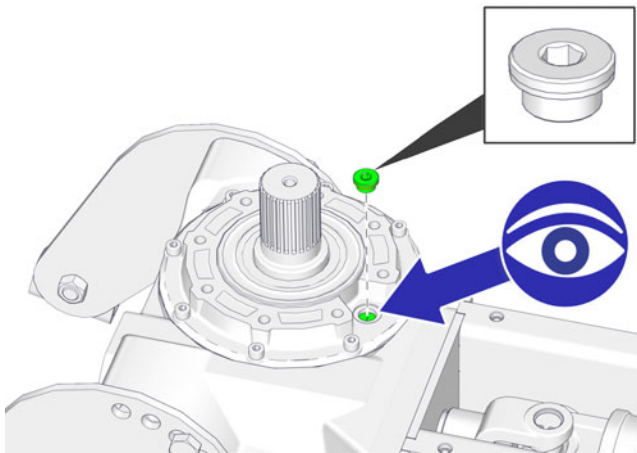
Fig. 7-2: Bouchon d'obturation
