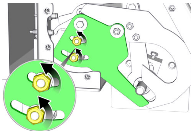
Fig. 8-17: Écrous
