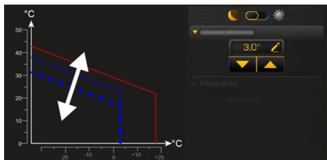
Fig. 6-102: Ajustement du fonctionnement de réduction
