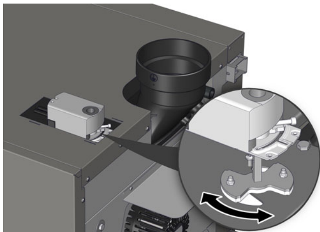
Fig. 4-1: Fonction de recyclage des fumées
