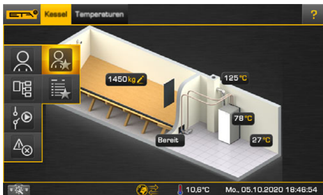
Fig. 6-47: Vue utilisateur
