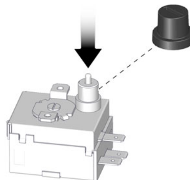
Fig. 3-2: Déverrouiller le contacteur de sécurité thermique
