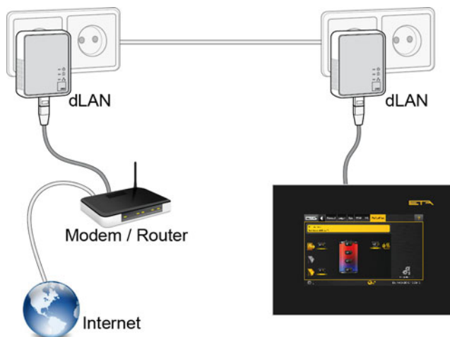
Fig. 6-33: Réseau dLAN
