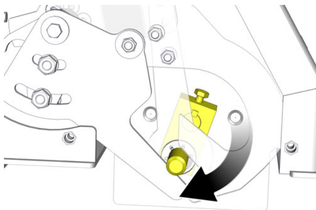
Fig. 8-15: Manivelle
