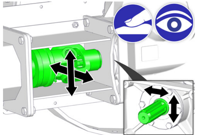
Fig. 7-3: Jeu au niveau du palier à l'entrée de la boîte de vitesses
