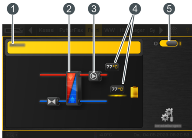
Fig. 6-119: Réseau comme station de transfert
