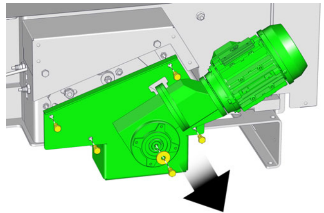
Fig. 8-13: Moteur
