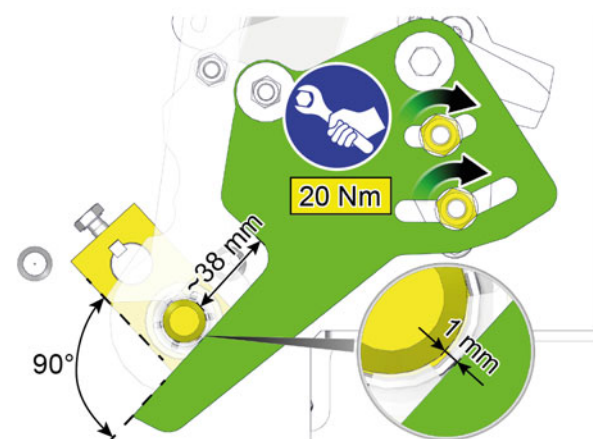
Fig. 8-19: Extraction à droite
