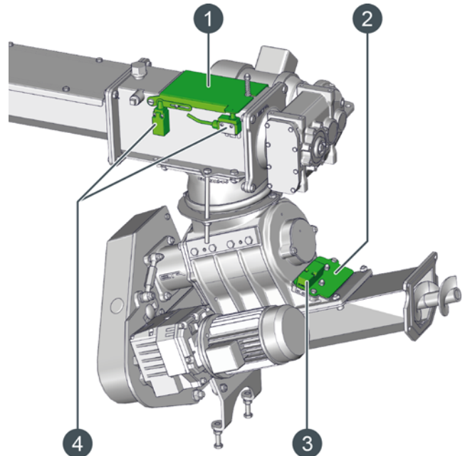
Fig. 8-1: Points d'accès pour l'élimination des blocages
